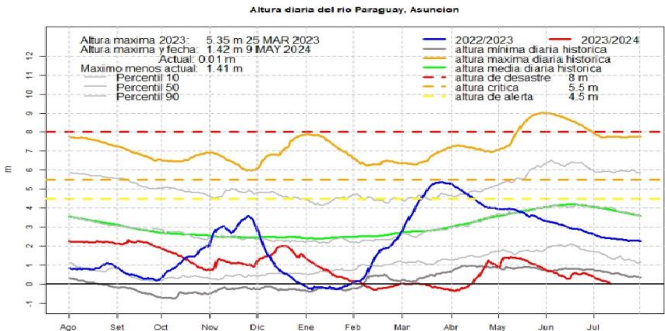
Figura I: Altura diaria del Río Paraguay, Puerto Asunción. Entre agosto-2023 y julio-2024
