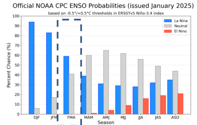
Figura 2. Probabilidad de fases del ENSO para la región de El Niño 3.4 actualizado al 9 de enero de 2025. Fuente: IRI (Instituto Internacional de Investigación para el Clima y La Sociedad).
